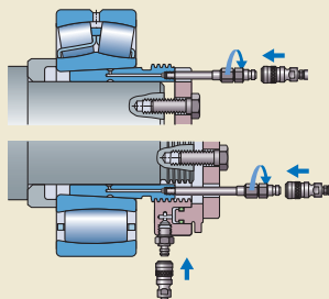
Bucha de desmontagem
