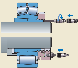
Bucha de fixação
