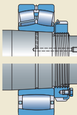
Eixo cônico
