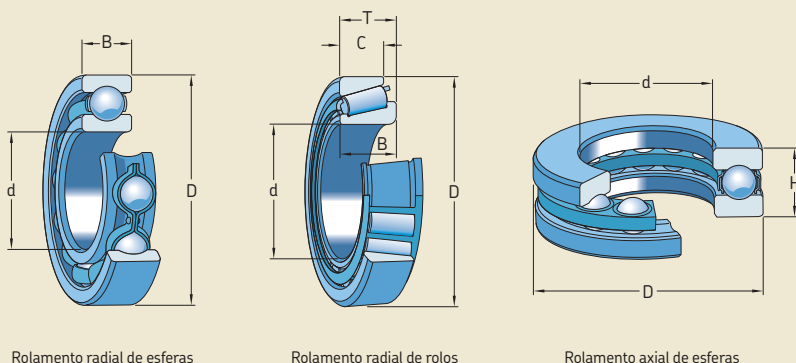
Rolamento radial de esferas
