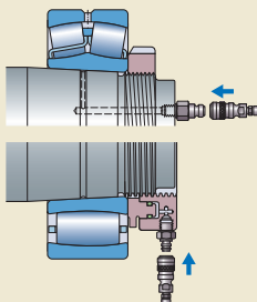
Eixo cônico
