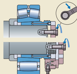
Bucha de desmontagem
